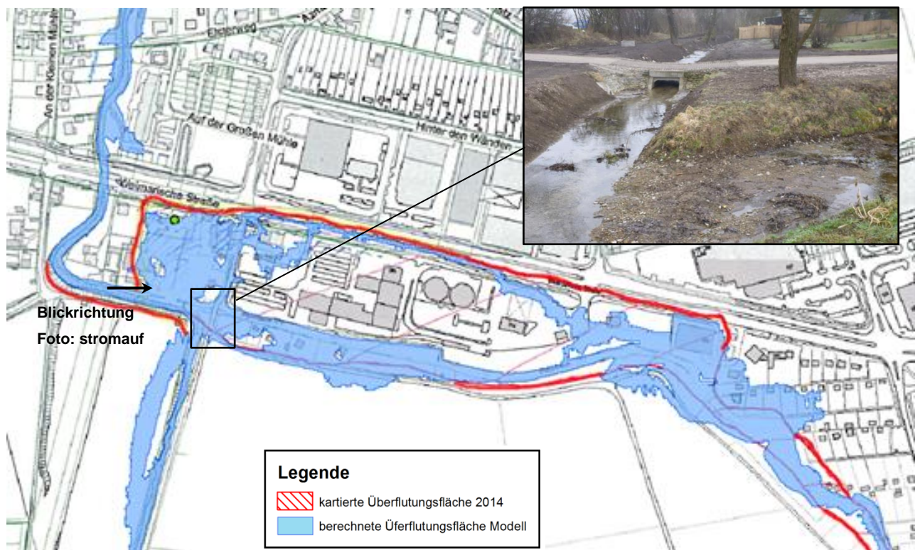
Abbildung 7-6 Linderbach Weimarische Straße, Hochwasser 2014 – Vergleich Kalibrierungsergebnis
