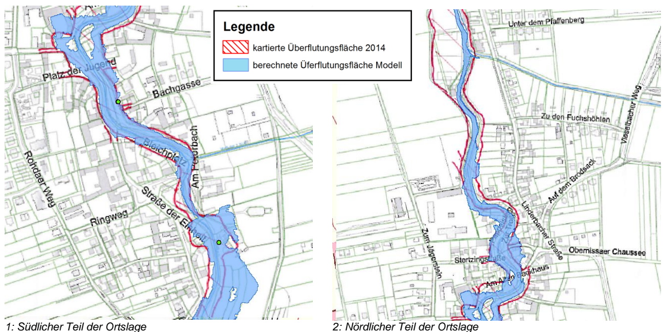
Abbildung 7-5 Büßleben, Hochwasser 2014 – Vergleich Kalibrierungsergebnis
