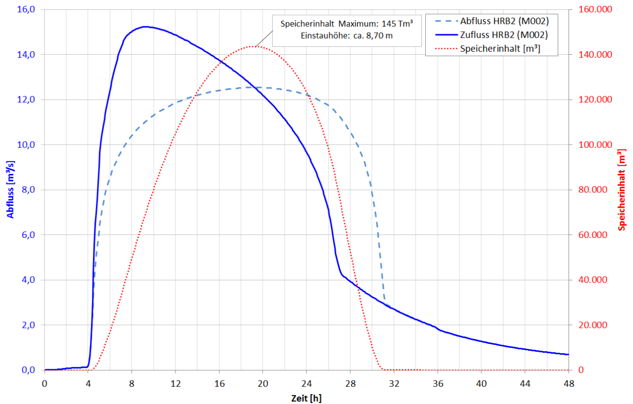
Abbildung 8-14 Variante 2: Ganglinien der Speichersimulation M002 – Becken uh. Rohda
