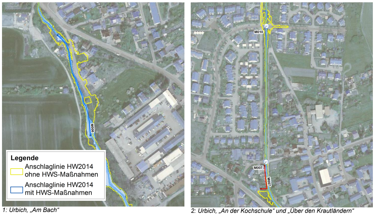
Abbildung 8-22 HW 2014 mit Hochwasserschutzmaßnahmen, Urbich
