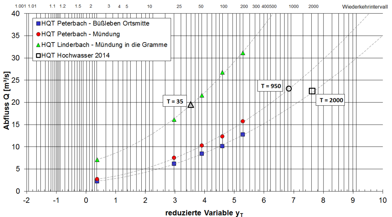
Abbildung 7-19 Wahrscheinlichkeit HQ_T -Ereignisse an ausgewählten Querschnitten (Gumbelverteilung)
