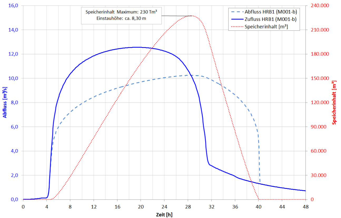
Abbildung 8-15 Variante 2: Ganglinien der Speichersimulation M001-b – Becken oh. Büßleben
