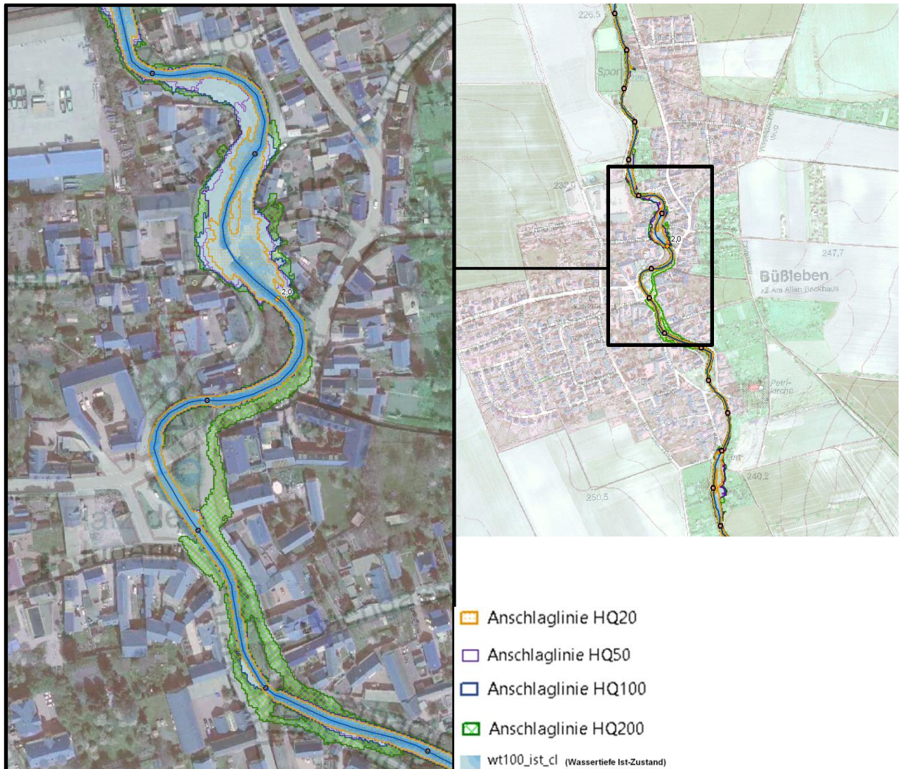
Abbildung 7-12 Ortslage Büßleben – Gewässer Peterbach, Flächenausbreitungen HQ 20 bis HQ 200
