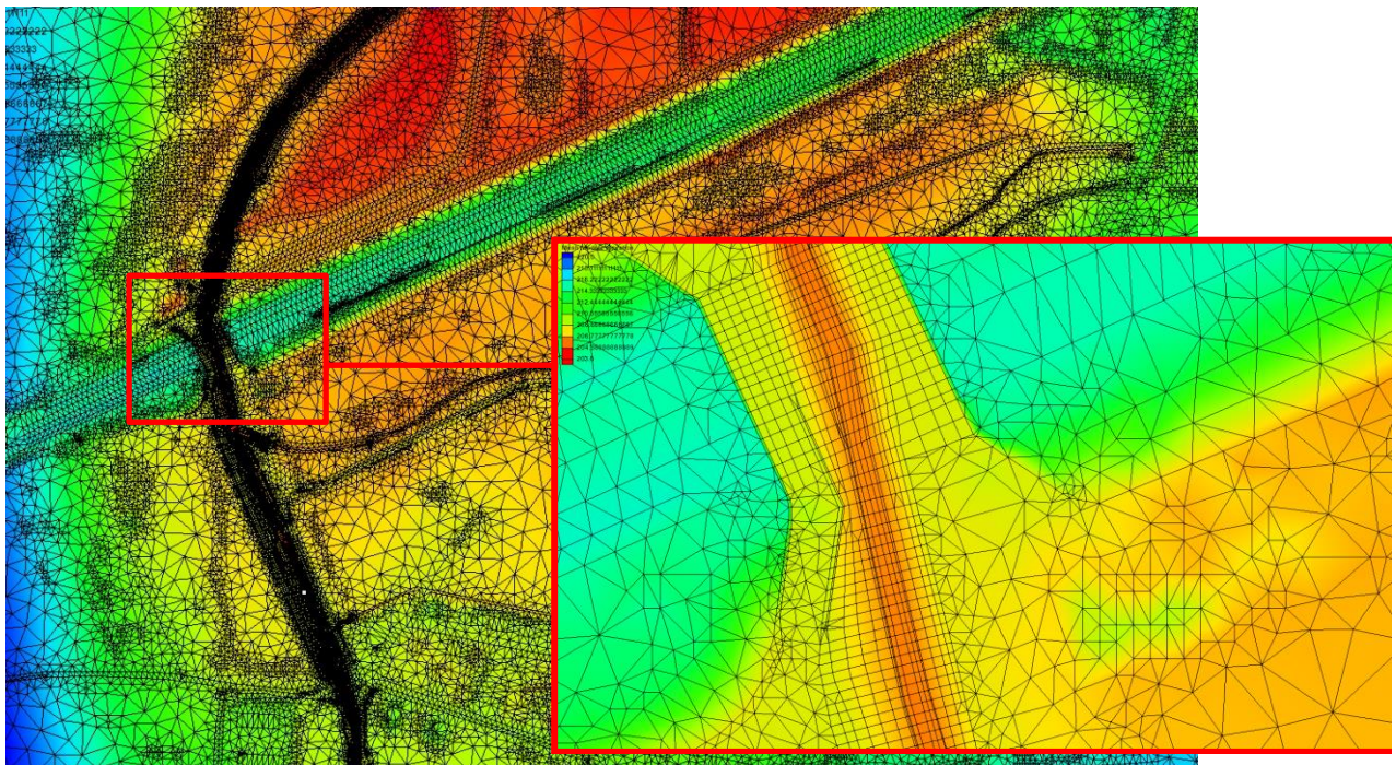
Abbildung 7-2 Ausschnitt aus dem 2D-Modellnetz (Querung Linderbach – Bahnstrecke)
