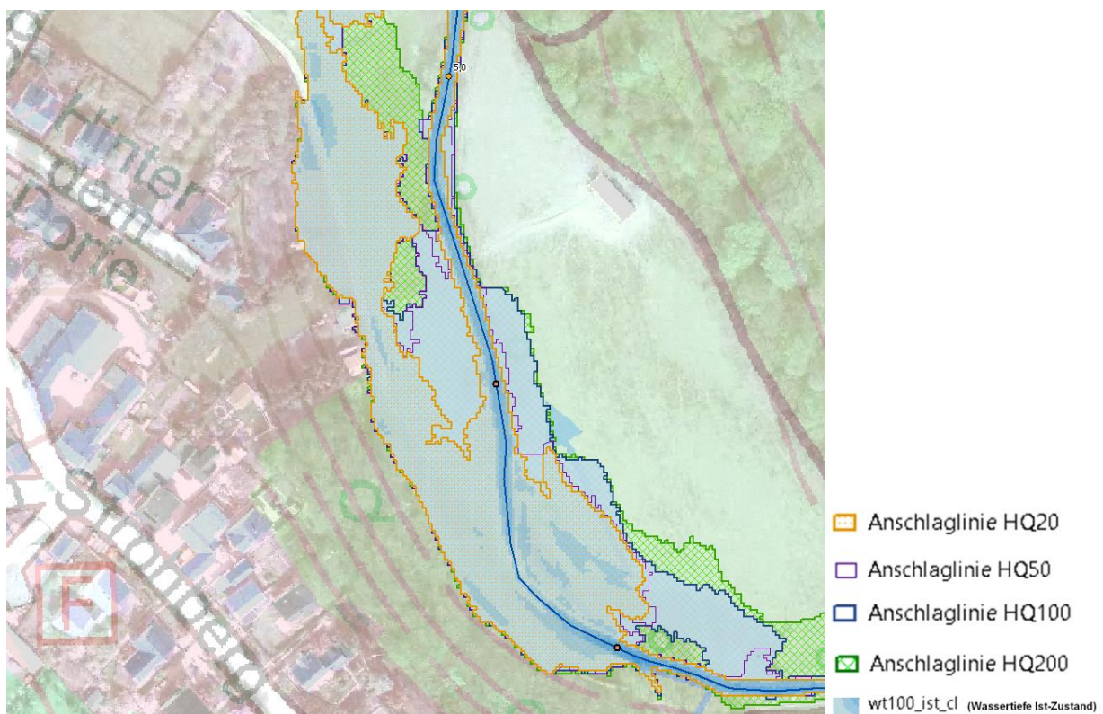
Abbildung 7-11 Ortslage Rohda – Gewässer Peterbach, Flächenausbreitungen HQ_{20} bis HQ_{200}
