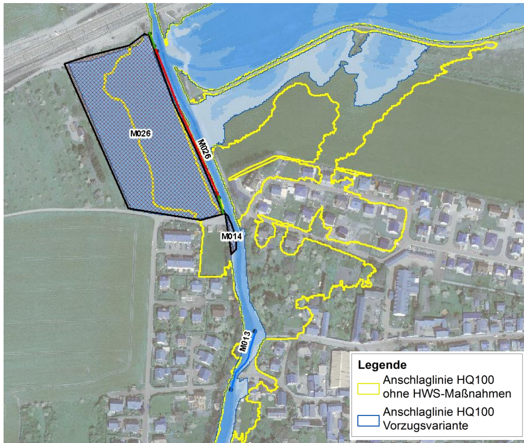
Abbildung 8-6 Ortslage Linderbach - Auswirkungen der Maßnahmen M013, M014 und M026
