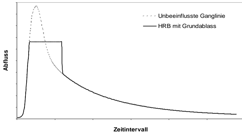
Abbildung 8-10 Wirkung eines HRB mit konstanter Abgabe über Grundablass (vereinfacht)
