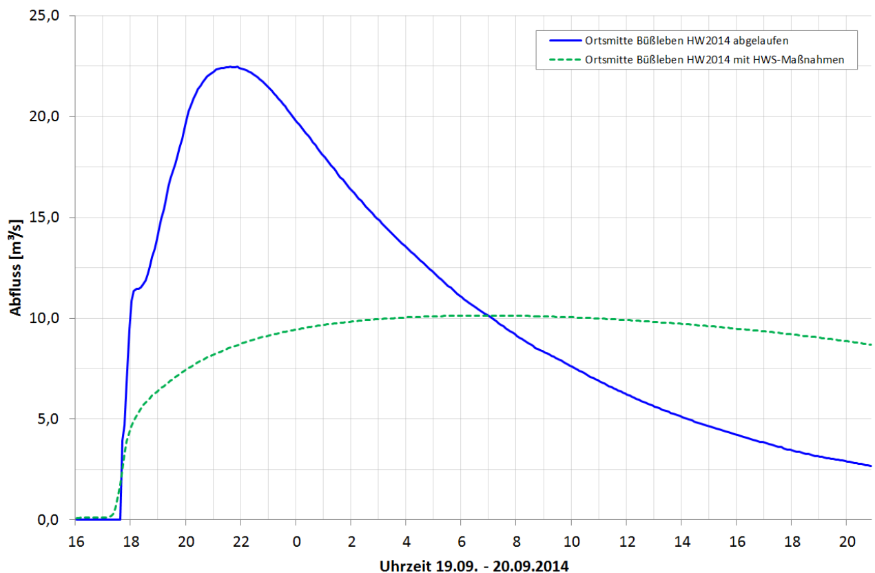
Abbildung 8-19 HW 2014 Abflussganglinie Büßleben - abgelaufen und prognostiziert
