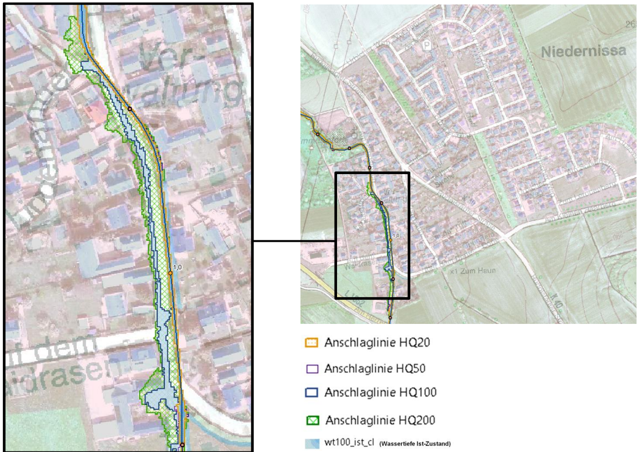
Abbildung 7-13 Ortslage Niedernissa – Gewässer Pfingstbach, Flächenausbreitungen HQ 20 bis HQ 200
