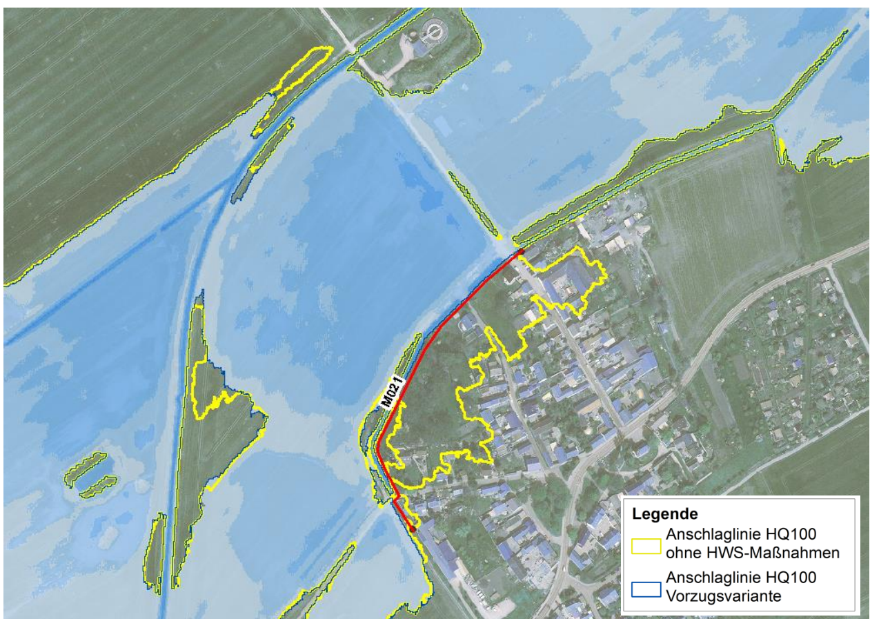
Abbildung 8-8 Ortslage Töttleben - Auswirkungen der Maßnahmen M016, M017, M019 und M020
