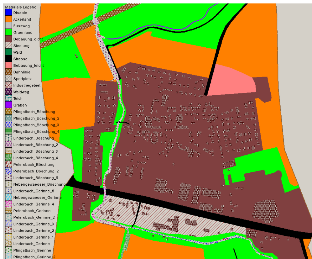
Abbildung 7-3 Rauheitsbelegung des 2D-Modells
