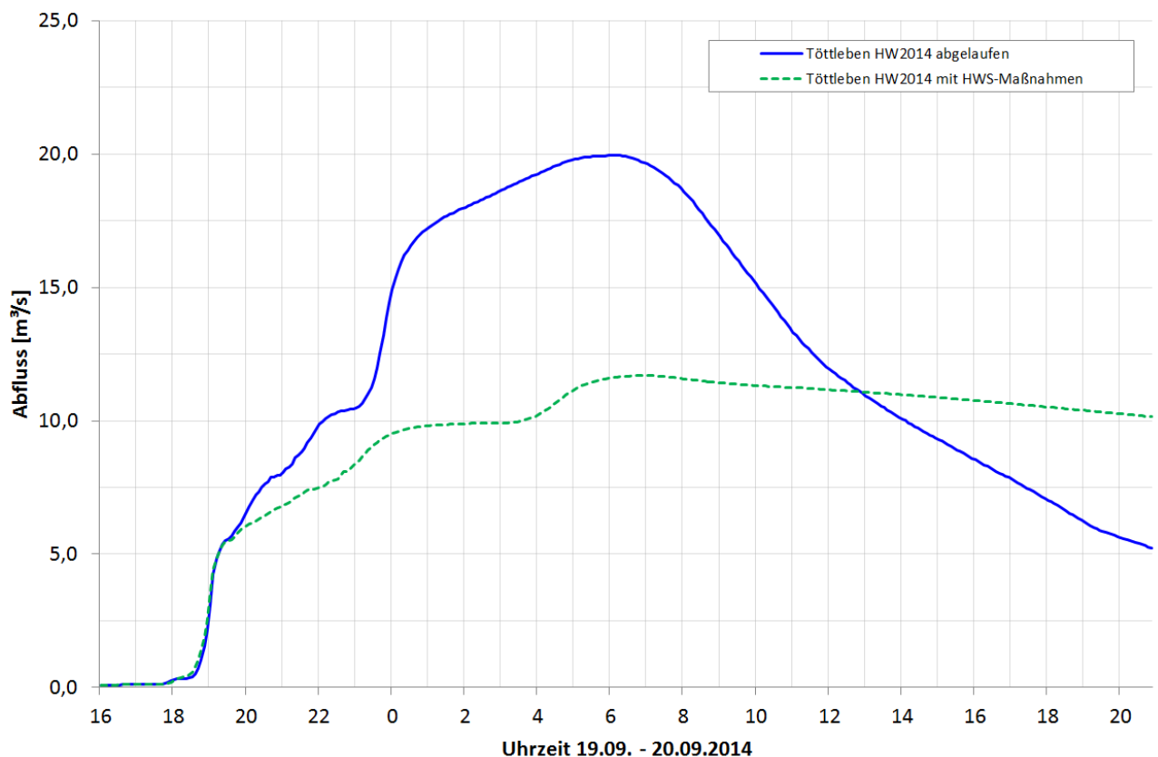
Abbildung 8-25 HW 2014 Abflussganglinie Töttleben - abgelaufen und prognostiziert
