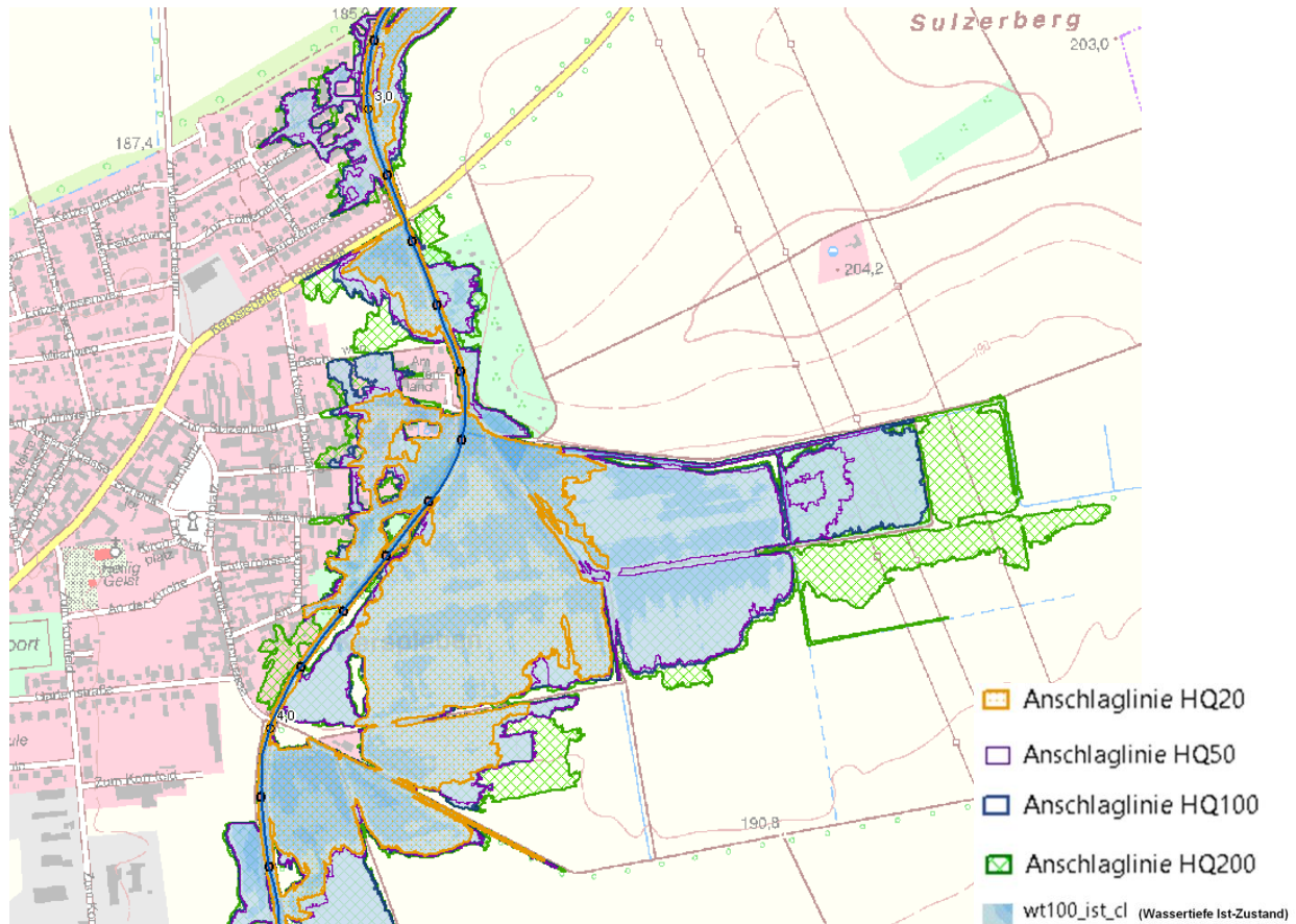
Abbildung 7-17 Ortslage Kerspleben, Gewässer Linderbach – Flächenausbreitungen HQ 20 bis HQ 200
