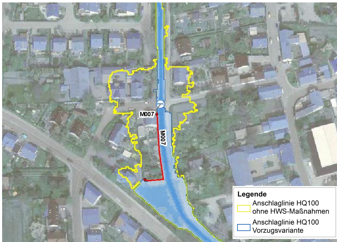
Abbildung 8-5 Auswirkungen der Maßnahme M007 in Urbich
