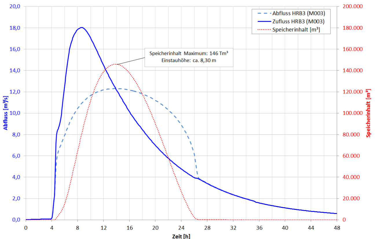
Abbildung 8-13 Variante 2: Ganglinien der Speichersimulation M003 – Becken oh. Rohda
