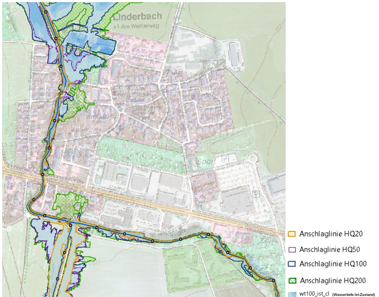
Abbildung 7-15 Ortslage Linderbach – Flächenausbreitungen HQ 20 bis HQ 200
