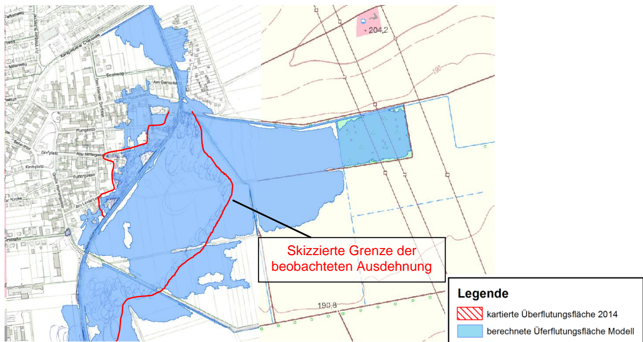
Abbildung 7-9 Kerspleben, Hochwasser 2014 – Vergleich Kalibrierungsergebnis
