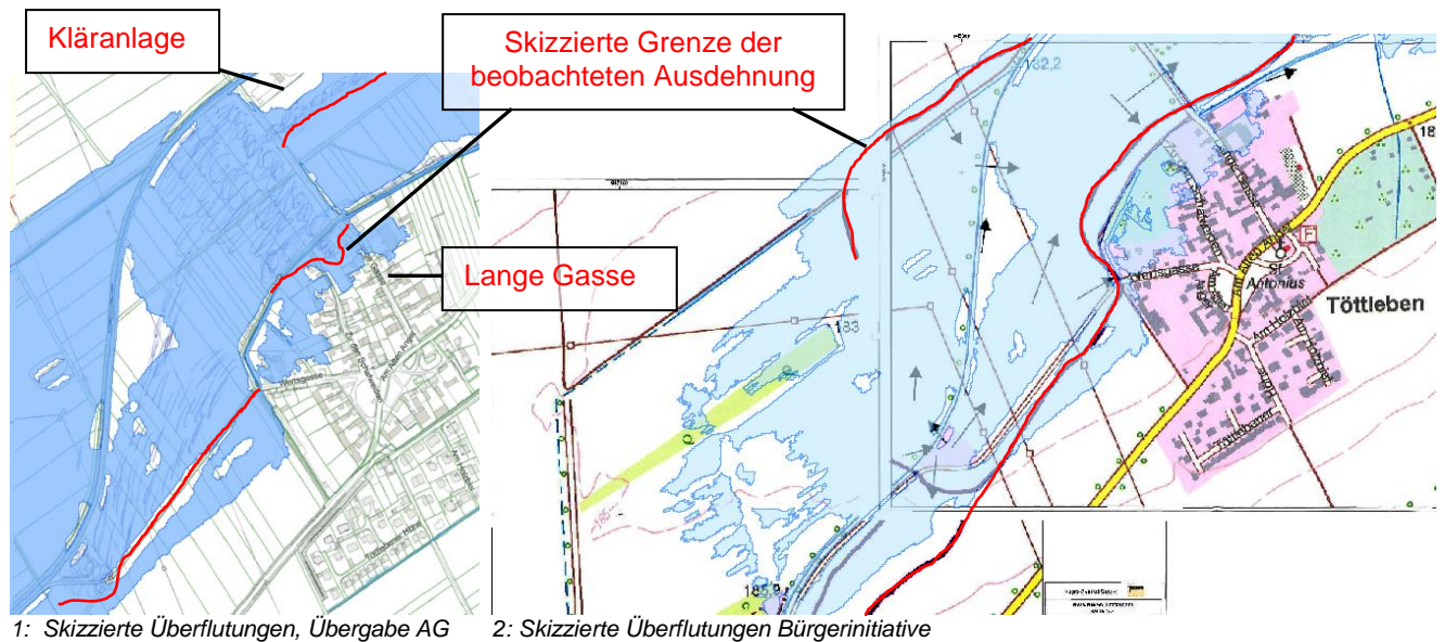
Abbildung 7-10 Töttleben, Hochwasser 2014 – Vergleich Kalibrierungsergebnis
