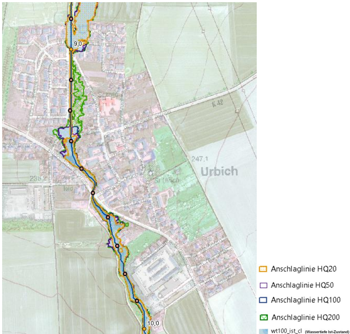
Abbildung 7-14 Ortslage Urbich – Gewässer Urbach, Flächenausbreitungen HQ 20 bis HQ 200
