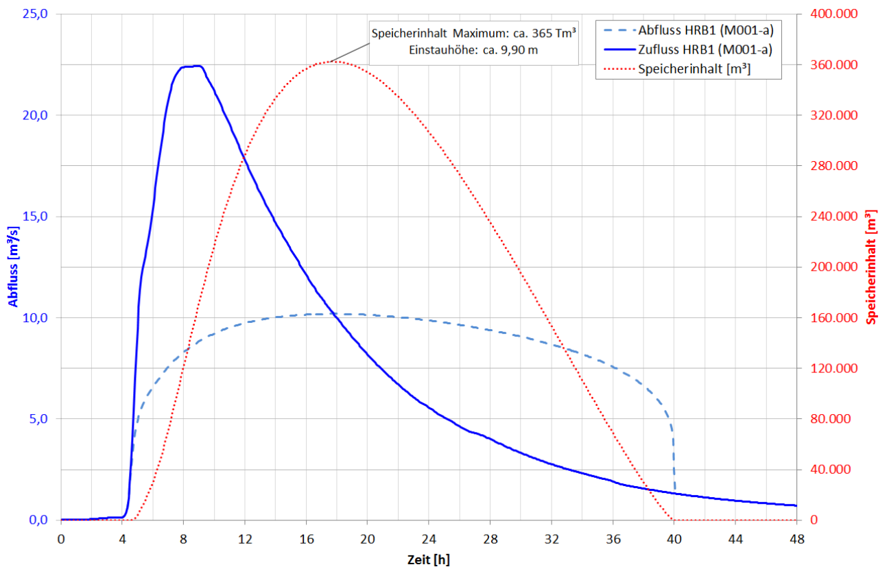
Abbildung 8-12 Variante 1: Ganglinien der Speichersimulation
