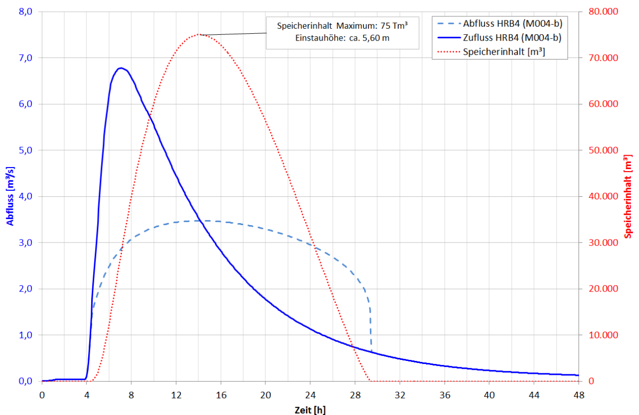
Abbildung 8-16 Variante 3: Ganglinien der Speichersimulation
