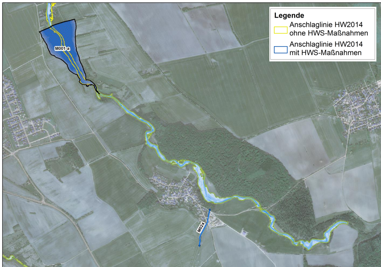
Abbildung 8-17 HW 2014 mit Hochwasserschutzmaßnahmen, oberhalb Büßleben
