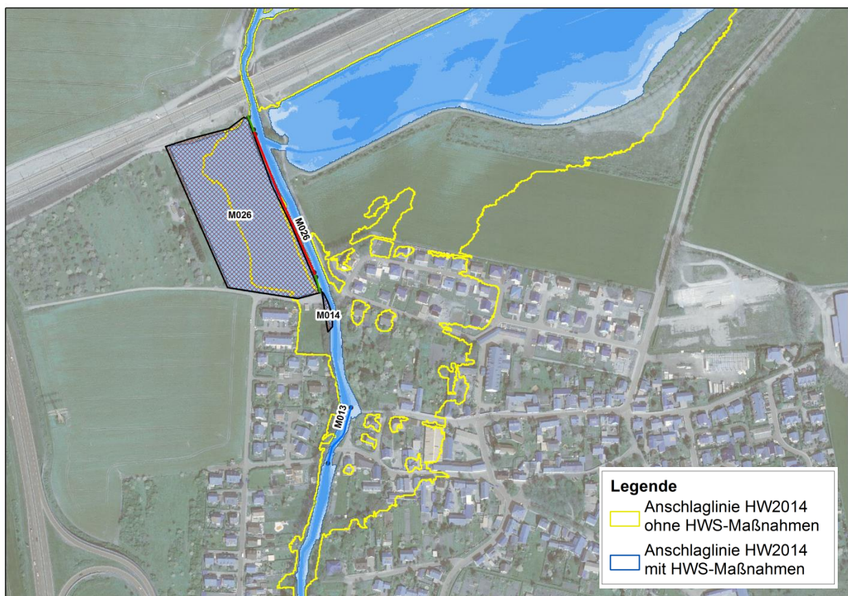
Abbildung 8-23 HW 2014 mit Hochwasserschutzmaßnahmen, Ortslage Linderbach
