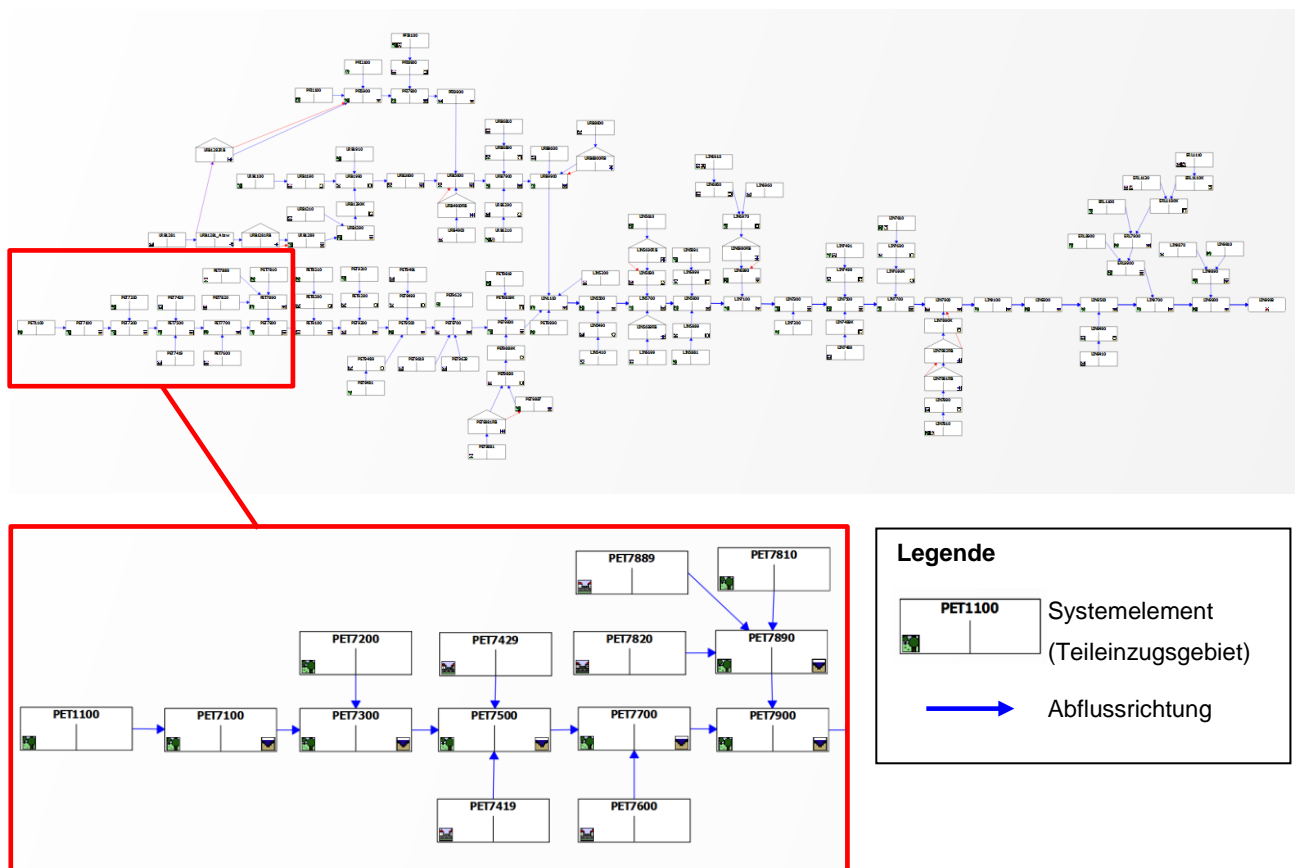
Abbildung 6-4 NASIM-Systemplan Linderbach
