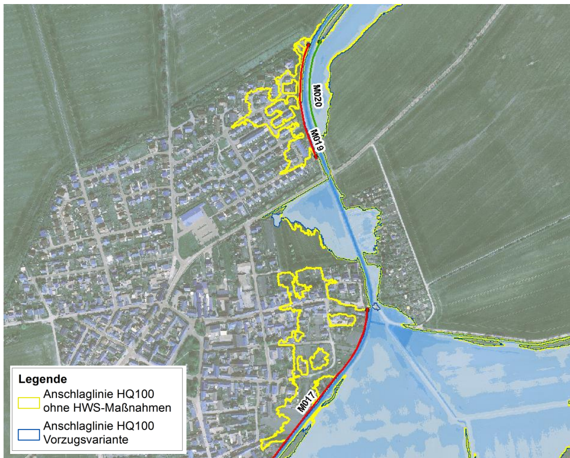
Abbildung 8-7 Ortslage Kerspleben - Auswirkungen der Maßnahmen M016, M017, M019 und M020
