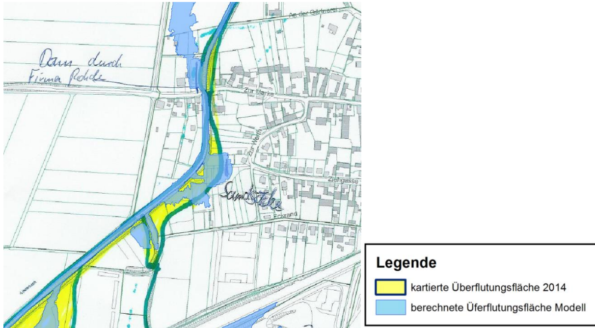
Abbildung 7-8 Azmannsdorf, Hochwasser 2014 – Vergleich Kalibrierungsergebnis
