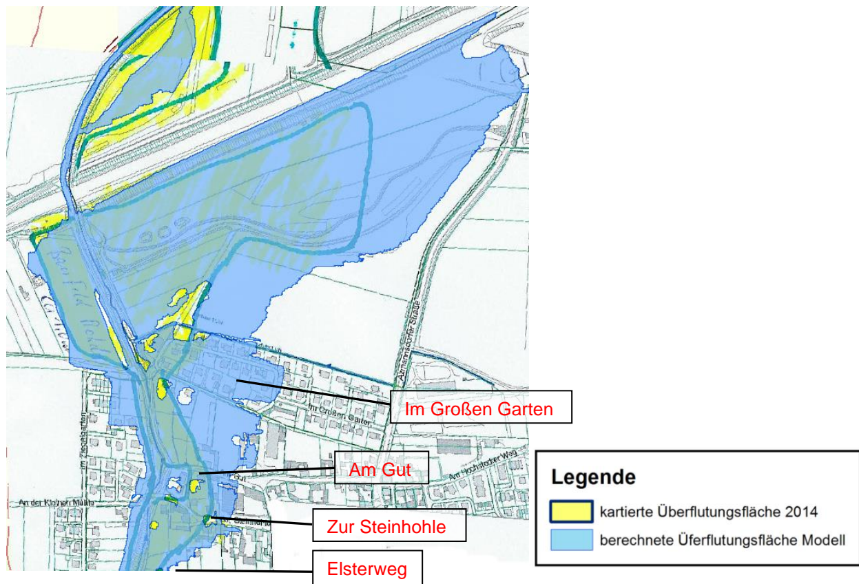
Abbildung 7-7 Linderbach, Ortsteil bis Bahnlinie, Hochwasser 2014 – Vergleich Kalibrierungsergebnis
