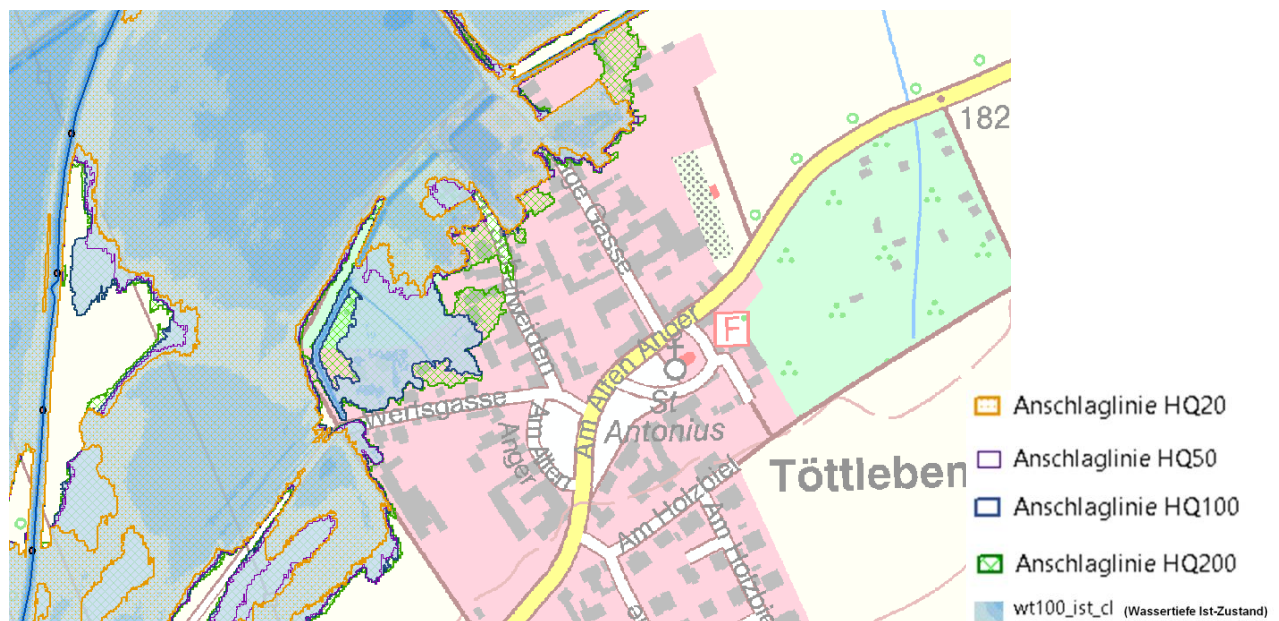
Abbildung 7-18 Ortslage Töttleben, Gewässer Linderbach – Flächenausbreitungen HQ 20 bis HQ 200
